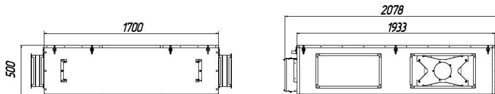
Рис 10. Габаритные размеры SlimStar 2000
